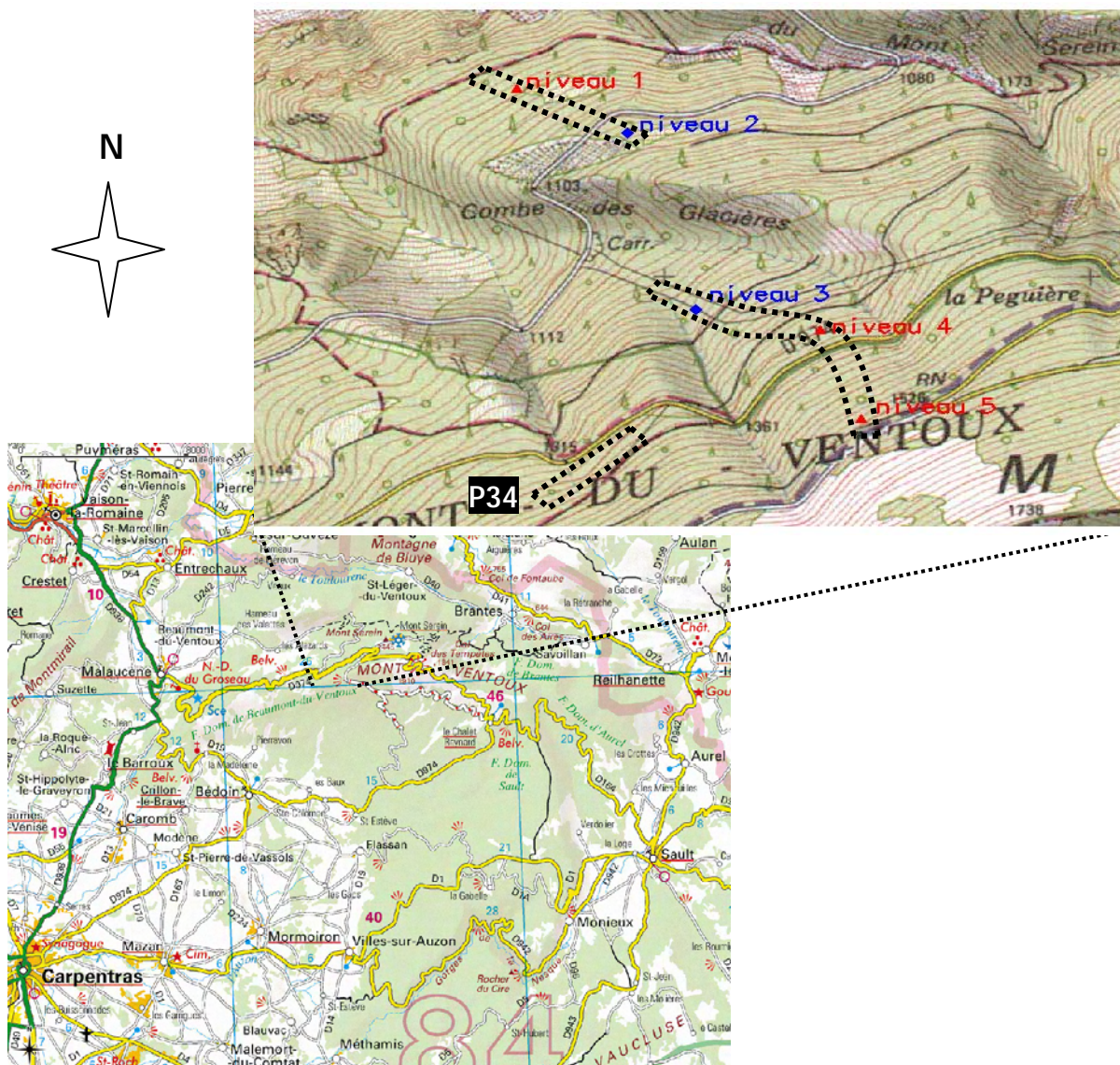
Figure a : Localisation du gradient Nord et de la parcelle 34 du Mont-Ventoux
