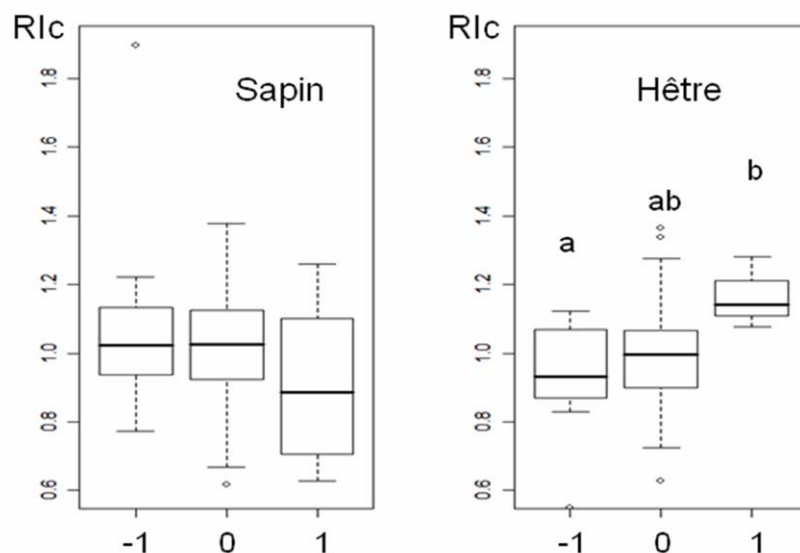
Figure 5 : Impact de la date de débourrement végétatif sur la croissance des sapins et des hêtres. En abscisse : la classe -1 correspond aux arbres qui ont débourré en avance d'au moins 4 jours par rapport aux arbres de même niveau altitudinal. La classe 1 correspond aux arbres en retard de 4 jours au minimum. En ordonnée, Rlc correspond pour chaque classe, à la moyenne des rapports entre les indices de croissance individuels et la moyenne des indices de croissance des arbres de même groupe altitudinal. a est différent de b au seuil de significativité de 1% (Test de Tukey).
