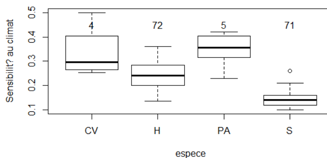
Figure 24: Etude de la variance de la sensibilité au climat
