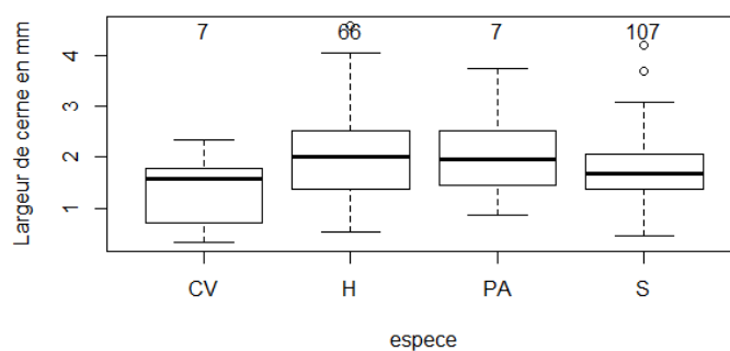
Figure 23: Etude de la variance de l'accroissement annuel
