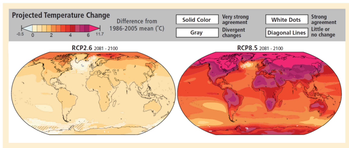
Figure 1: Prédiction sur l'évolution du climat d'ici 2100 (IPCC, 2014)
